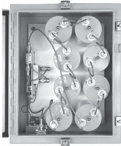
TTPA-3548 Tower Top Preamplifier/Preselector
