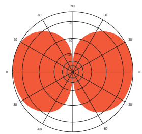
E-plane: 450 MHz
