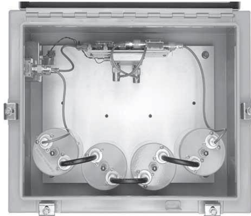
TTPA-4544 Towertop Preamplifier
